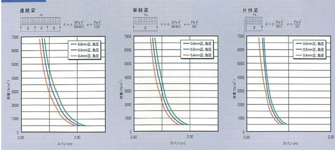
許容スパン
