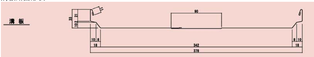
丸棧納め図
