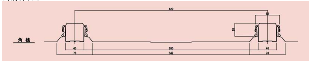
角棧納め図
